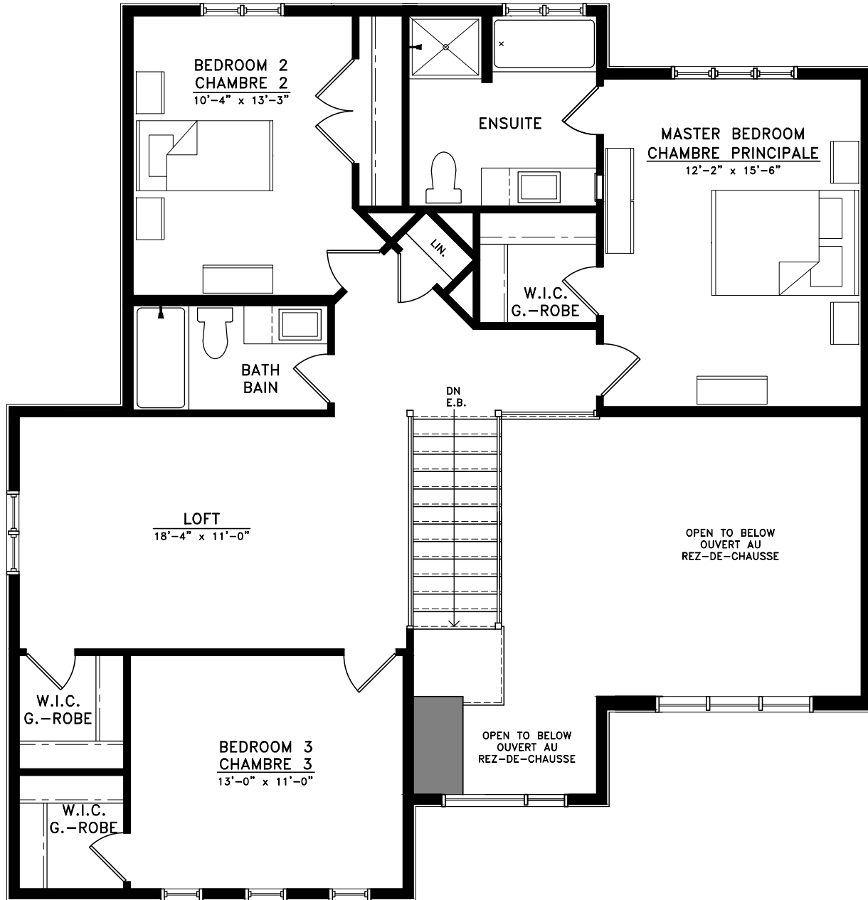
SECOND FLOOR PLAN / OPT. 3 BEDROOMS WITH LOFT 2ième PLANCHER / OPT. 3 CHAMBRES AVEC LOFT 1101 sq.ft. / pi2
