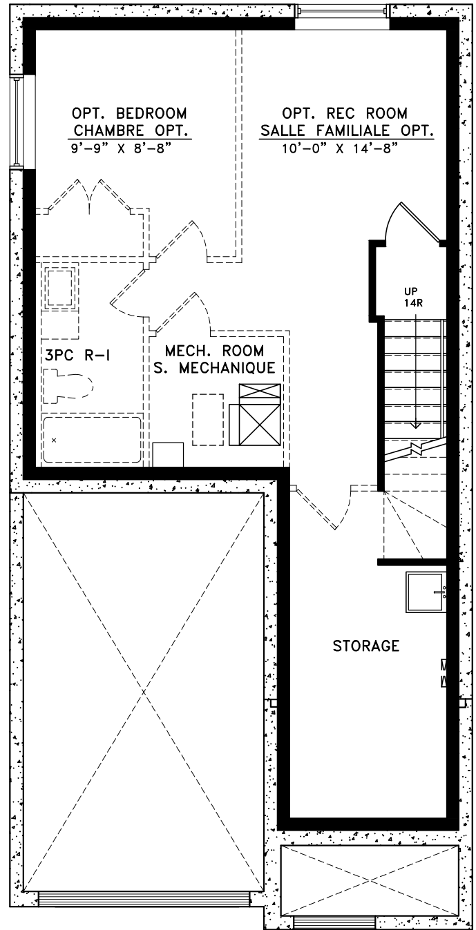
OPTIONAL FINISHED BASEMENT #2 SOUS-SOL FINI OPTIONNEL #2 15 sq.ft. / pi2
