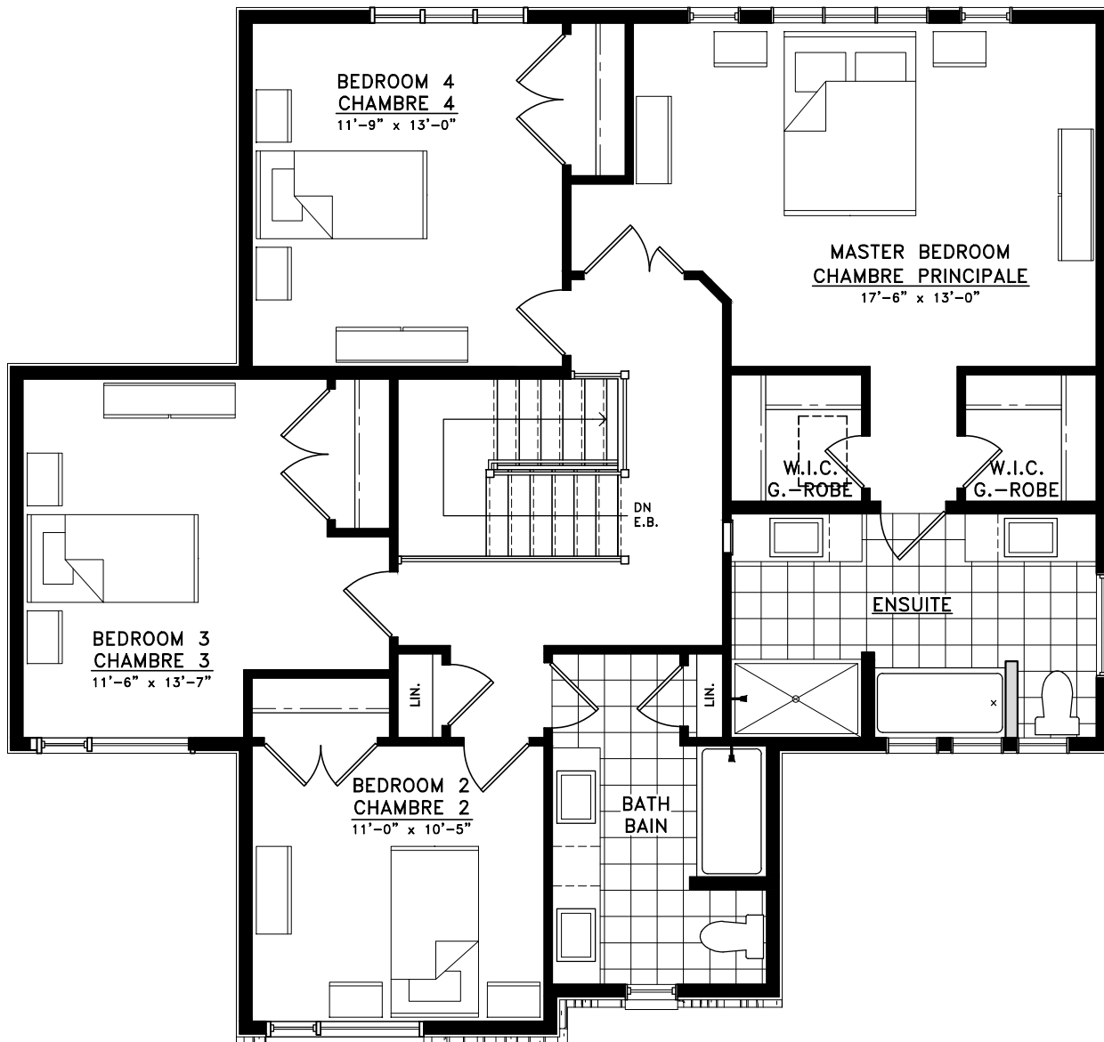
SECOND FLOOR PLAN / 4 BEDROOMS 2 ième PLANCHER / 4 CHAMBRES 1266 sq.ft. / pi2
